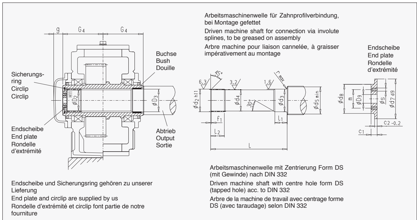
Bauarten / Types H2K., H3K., H4K., B3K., B4K.
